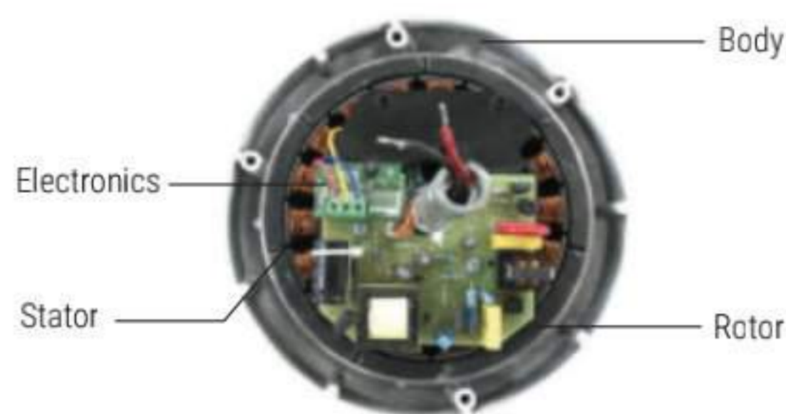
Atomberg Motor
